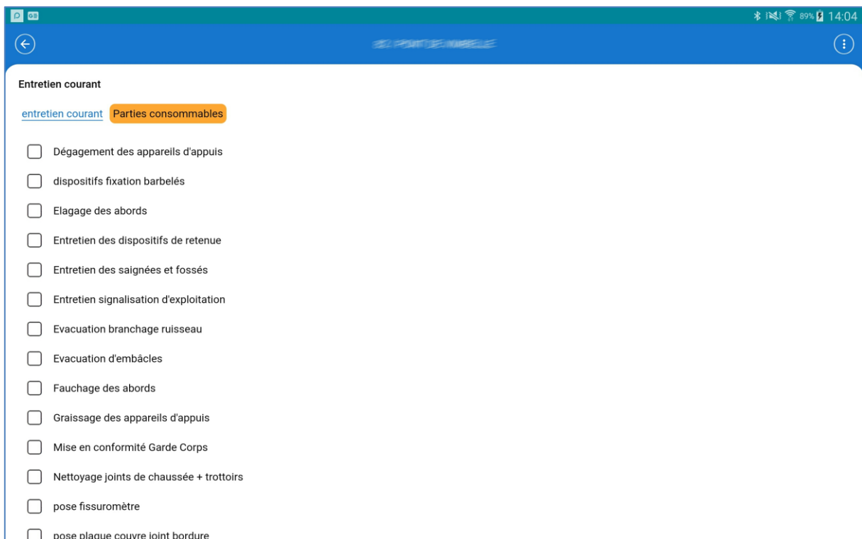
L'éditeur de demande d'entretien courant / Parties consommables
