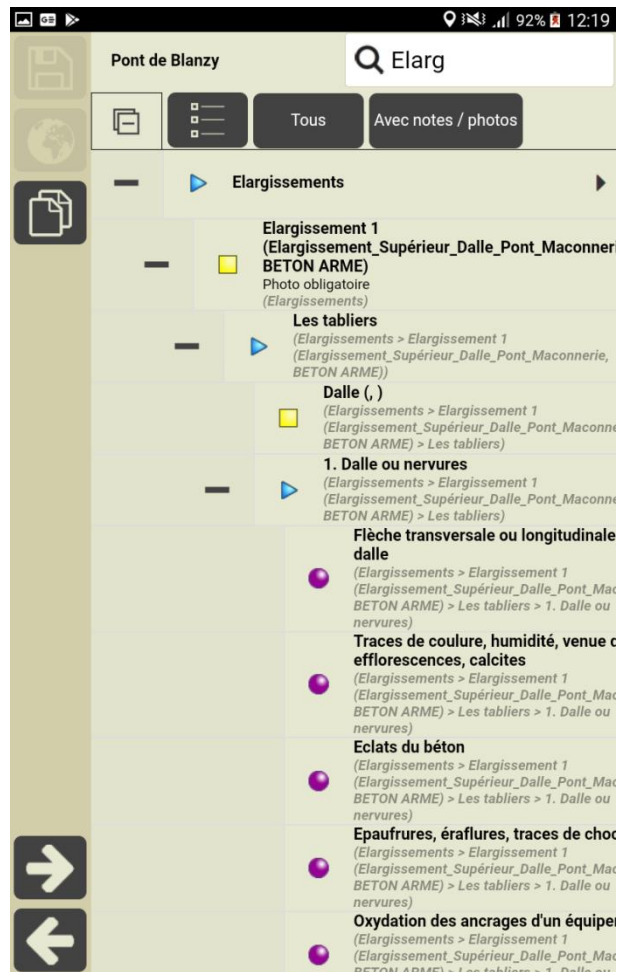
Pont de Blanzly : Elargissement supérieur Dalle Pont Maçonnerie
